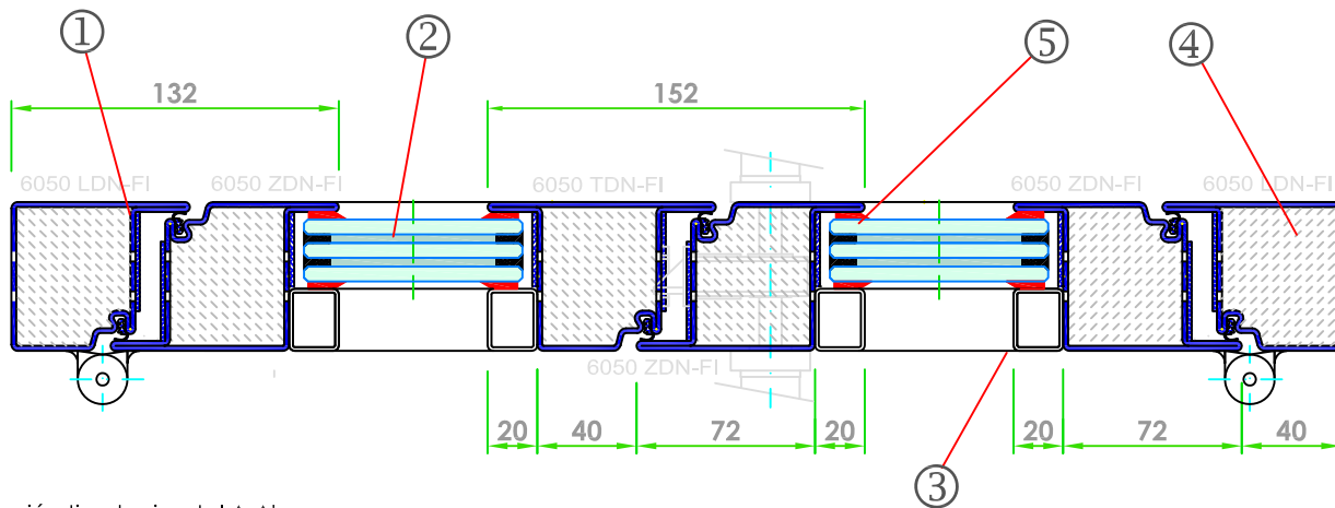
Sección tipo horizontal A-A' escala - 1:3
