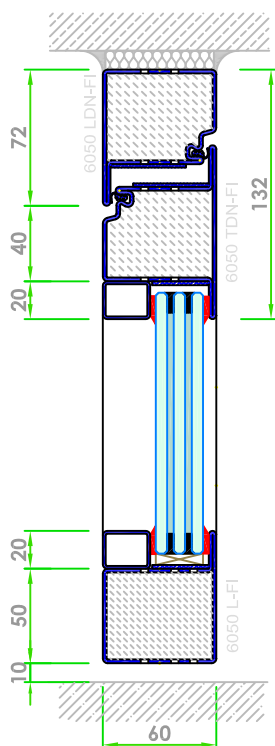
Sección tipo vertical B-B' escala: 1/4
